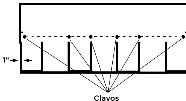
Clavado - Pendientes Pronunciadas o Con Viento Fuerte Se Requieren 6 Clavos
