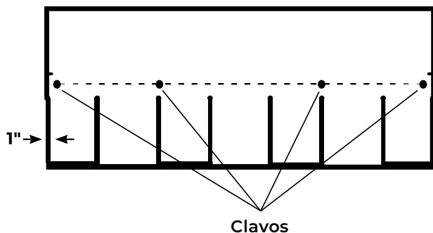
Aplicación Éstandar Se Requieren 4 Clavos
