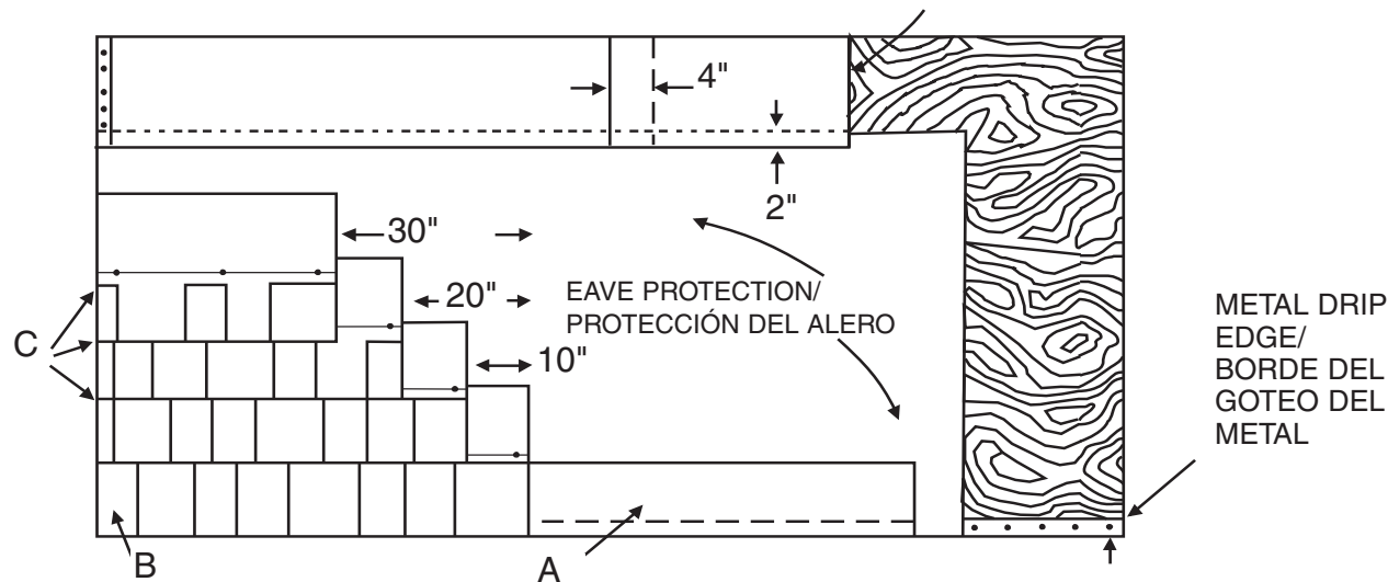
FIGURE 2: UNDERLAYMENT/CAPA INFERIOR DE RECUBRIMIENTO Y PROTECCIÓN PARA EL ALERO
